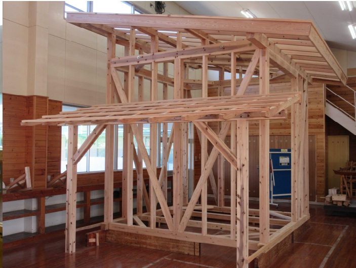
⑤木造倉庫（片流れ）
